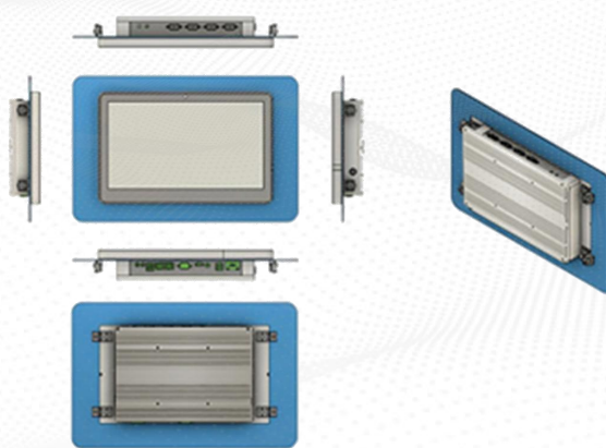
外嵌式安装
